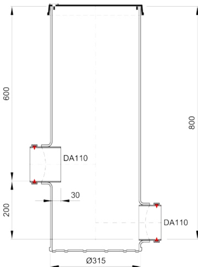
PVC - Probeentnahmeschacht DN 315 mit Gussdeckel A15, begehbar
