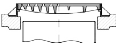
Gussabdeckung Klasse A15, B125 u. D400 mit Betonausgleichsring mit Z-Falz
